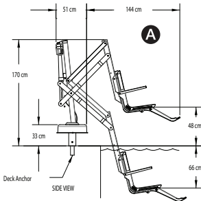
A SIDE VIEW VISTA LATERAL VUE DE CÔTÉ SEITENANSICHT YANDAN GÖRÜNÜM
