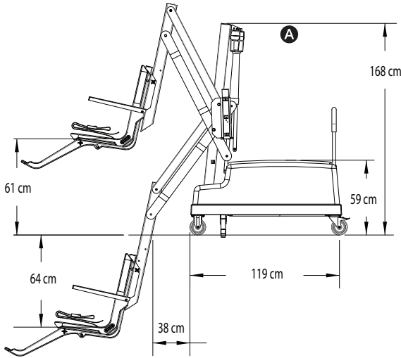
A SIDE VIEW VISTA LATERAL VUE DE CÔTÉ SEITENANSICHT YANDAN GÖRÜNÜM
