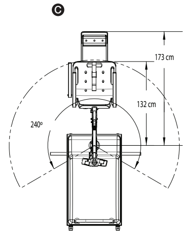
C TOP VIEW VISTA SUPERIOR VUE DE DESSUS DRAUFSICHT ÜSTTEN GÖRÜNÜM
