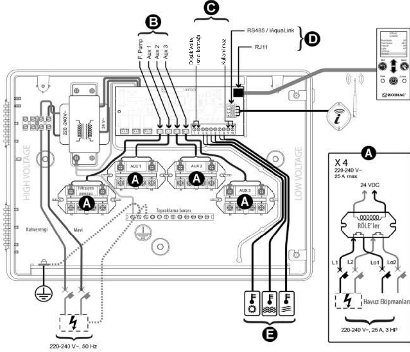
AquaLink® TRi standart bağlantı diyagramı
