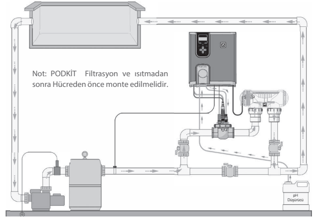
POD Kit by-pass şeması:
