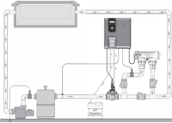
Hat üzeri POD Kiti:
