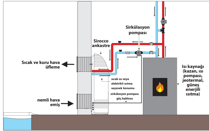
Sıcak su ısıtmalı olan bir cihazın montajı
