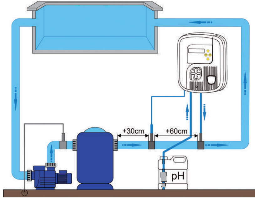
pH Clever MONTAJ diagram:
