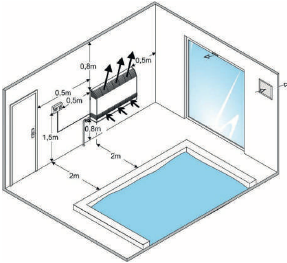
SIROCCO mahal model nem alma cihazının montaj örneği
