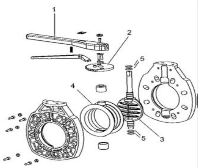
D63 - D225
